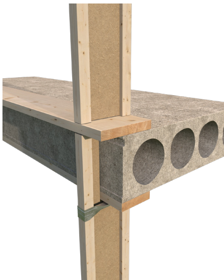
Exempellösning utfackningsvägg Monterad med urtag
