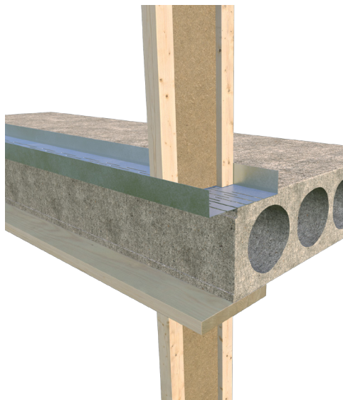
Exempellösning utfackningsvägg Monterad med vanlig syll och stålsyll
